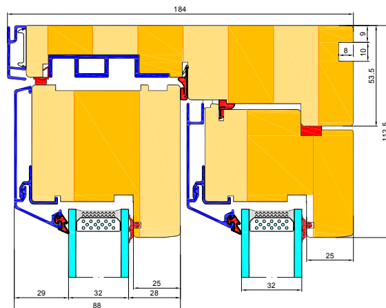
ECO LINE ALU _ szyba 32 mm
