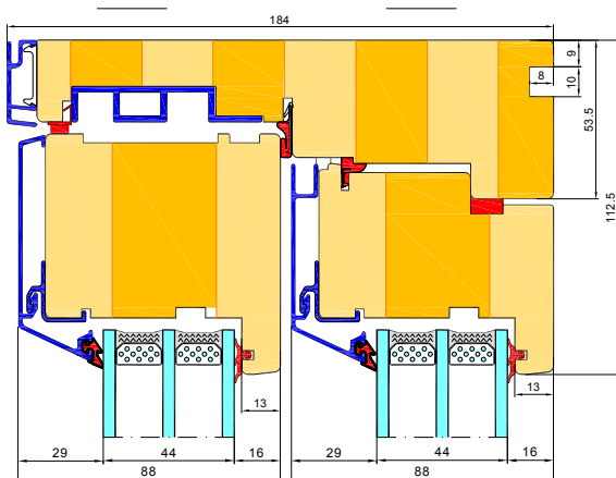
ECO LINE ALU _ szyba 44mm
