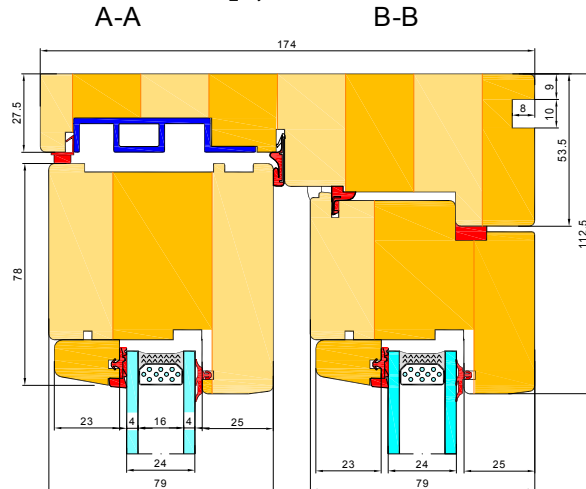
ECO LINE _ szyba 24 mm
