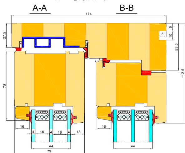
ECO LINE _ szyba 36mm, 44mm
