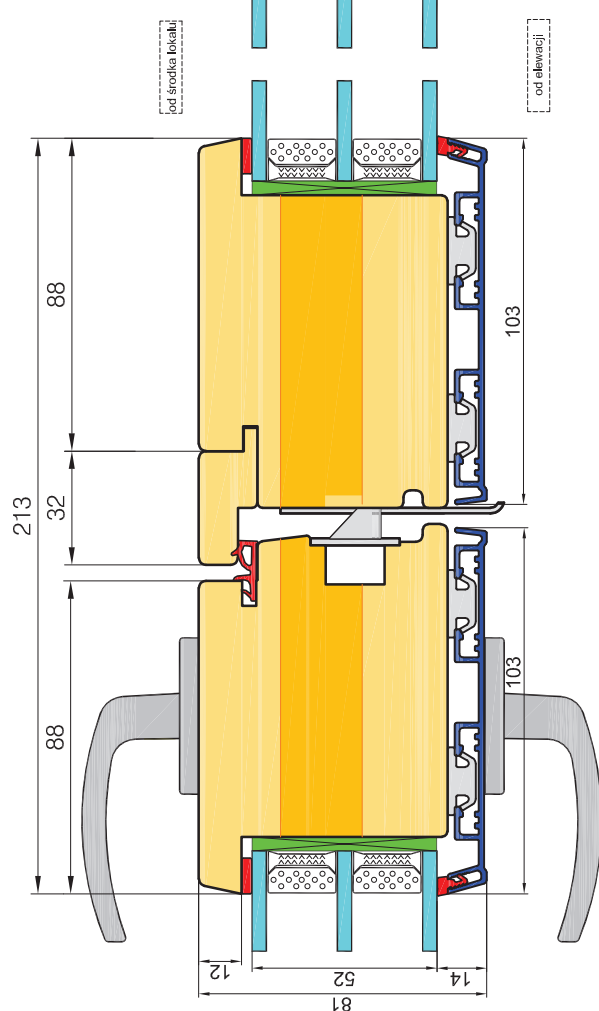
DRZWI OTWIERANE NA ZEWNAŁRZ - SŁUPEK RUCHOMY
