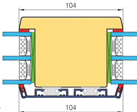
Szpros konstrukcyjny pionowy 104mm
