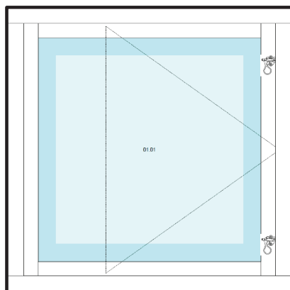
Side Swing (okucie OPTA-SG_90_A)
