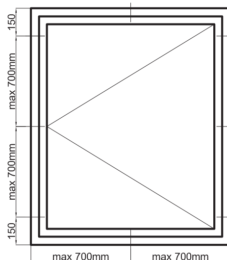
Rozmieszczenie nawierceń
