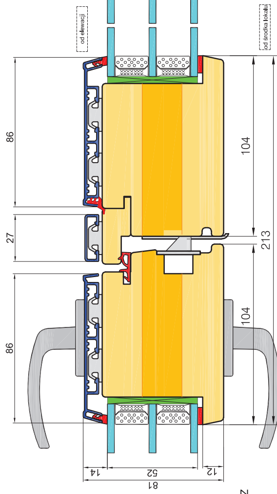
DRZWI OTWIERANE DO WĘWNAŁRZ - SŁUPEK RUCHOMY
