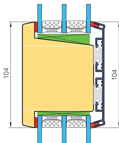
Szpros konstrukcyjny poziomy 104mm
