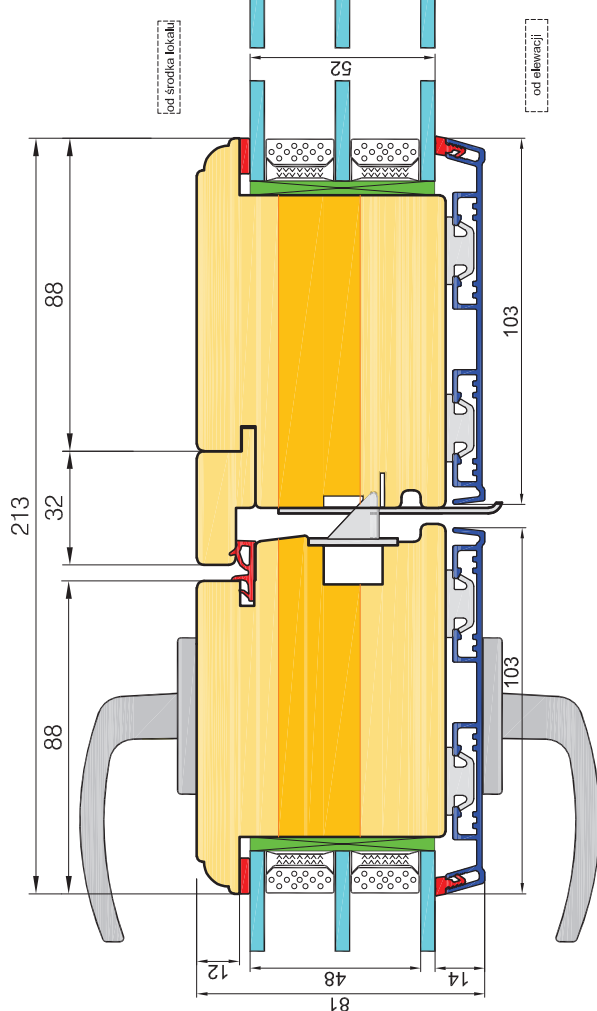
DRZWI OTWIERANE NA ZEWNĄTRZ - SŁUPEK RUCHOMY
