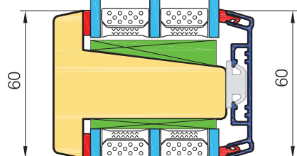
Szpros konstrukcyjny poziomy 60mm
