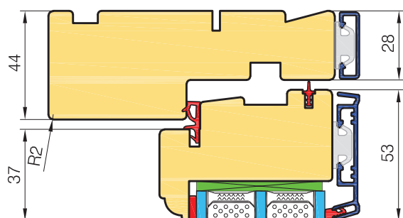
Szpros konstrukcyjny poziomy 60mm
